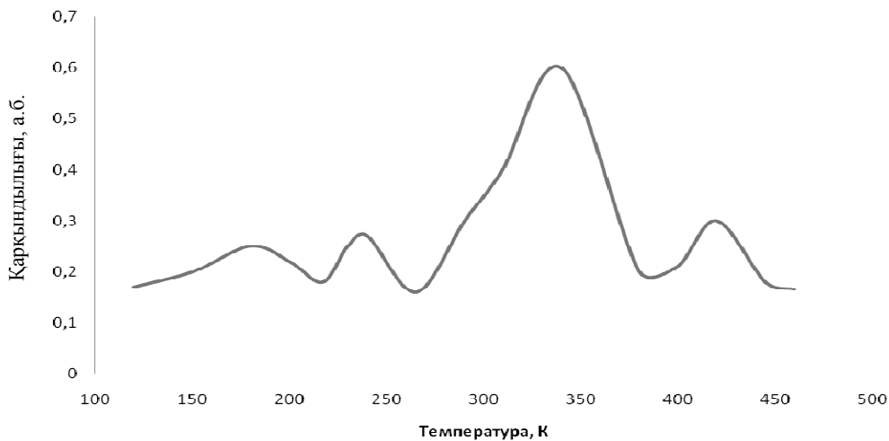
1-сурет. Сәулелендірілген K 2 SO 4 -Pb кристалының ТҚЛ
