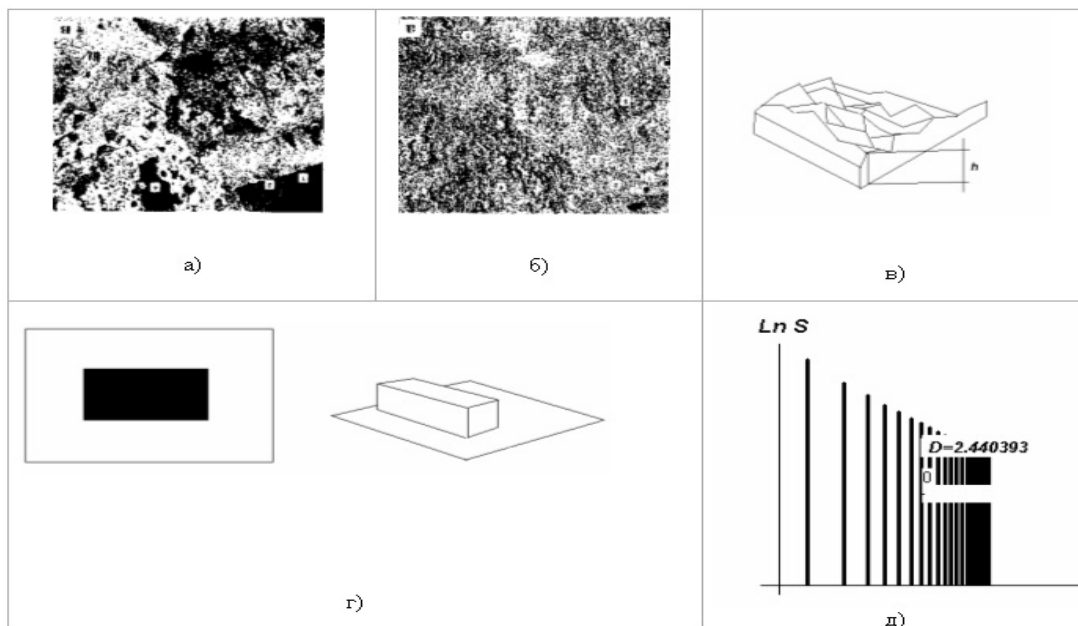
Рисунок 1. Примеры, объясняющие сущность фрактальной обработки (а-с), и фрактальная пространственная сигнатура (д)
