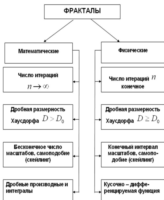
Рисунок 2. Авторская классификация фрактальных множеств и сигнатур
