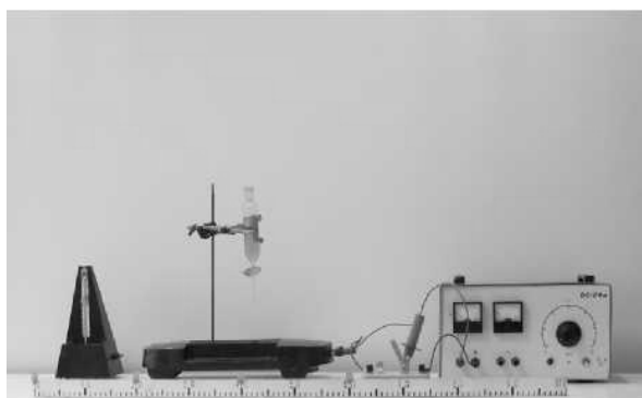
а — бірқалыпты қозғалыс тәжірибесінің дәстүрлі нұсқасы
